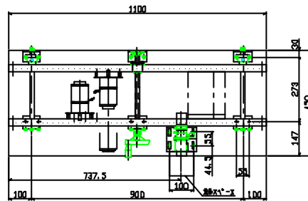
外形寸法図
