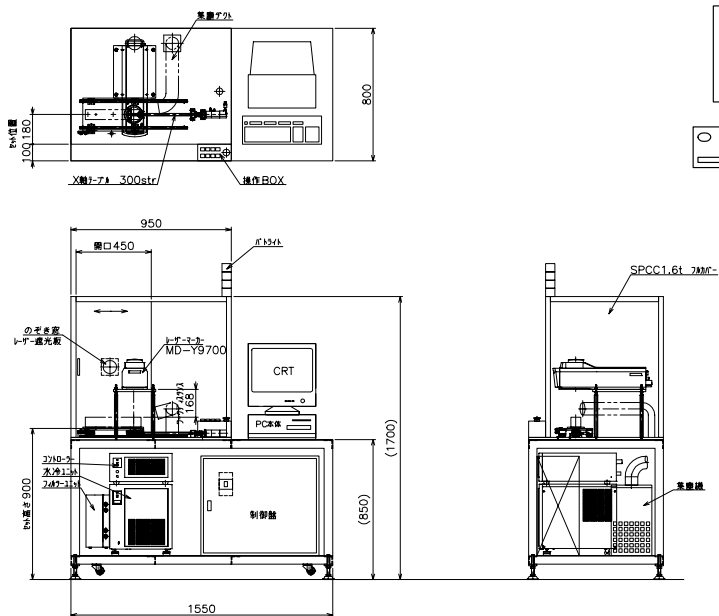
〈外形寸法図〉
